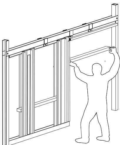
POSE DES 4 PROFILS SPECIFIQUES
